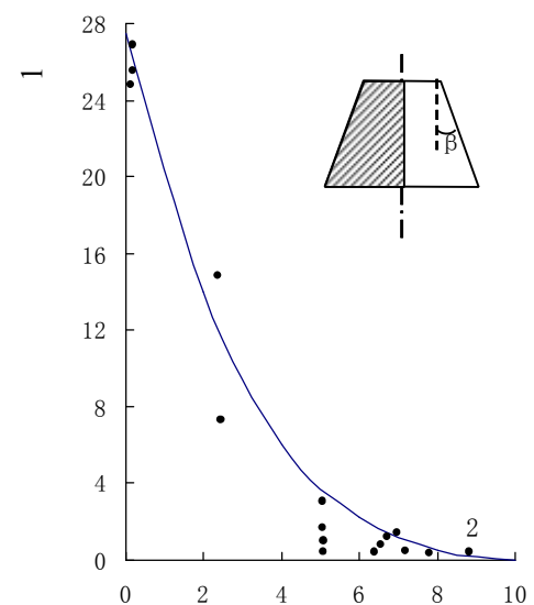
图2 斜面基础的抗冻拔试验
